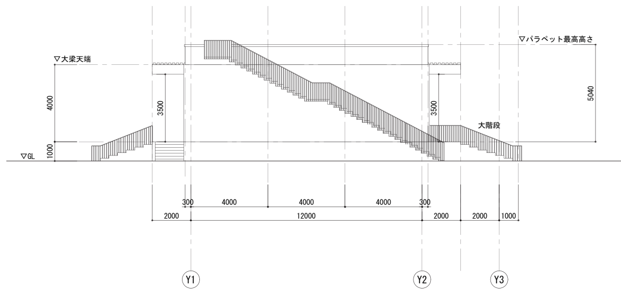
東立面図
