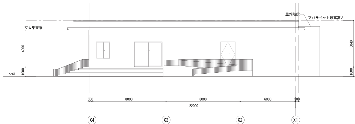
北立面図
