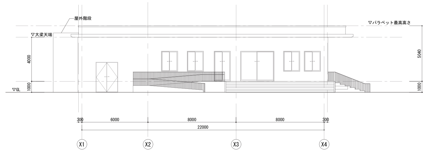
南立面図
