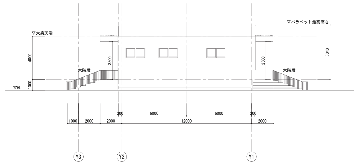
西立面図
