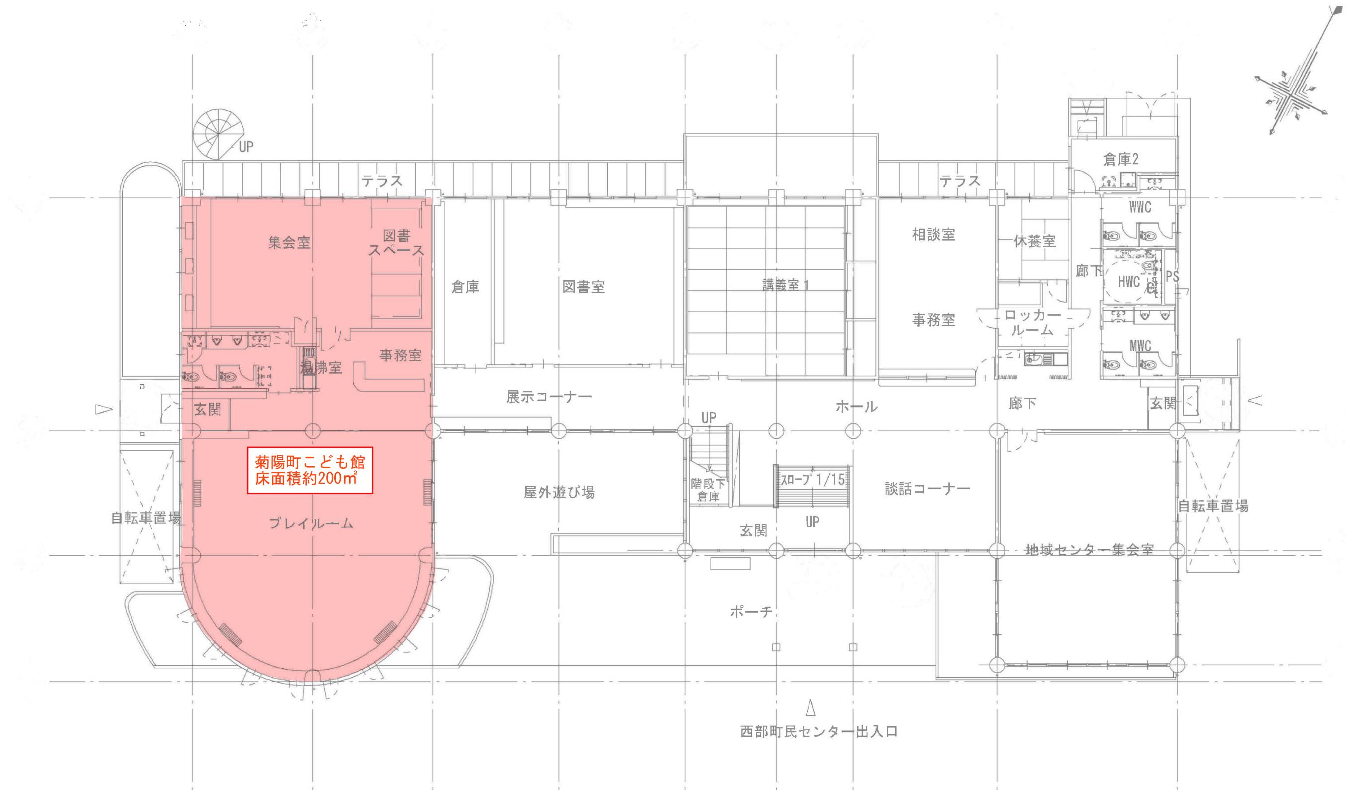
菊陽町西部町民センター平面図
